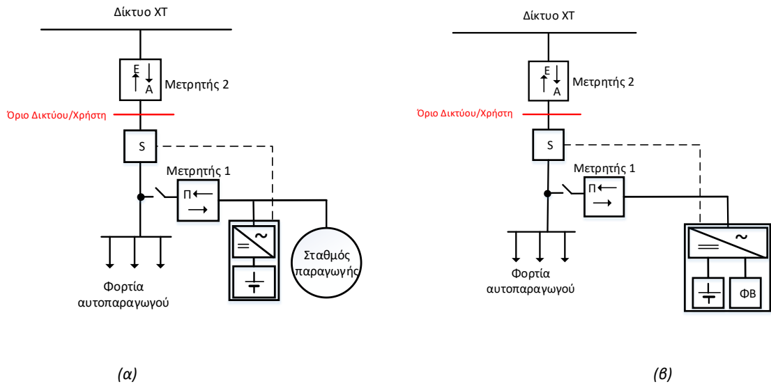
Σχήμα 1: Ενδεικτικό απλοποιημένο μονογραμμικό διάγραμμα εσωτερικής ηλεκτρικής εγκατάστασης ΧΤ όπως διαμορφώνεται α) μετά τη σύνδεση σταθμού παραγωγής και συσσωρευτών μέσω διαφορετικών μετατροπέων ( ac coupled ) και β) μετά τη σύνδεση ΦΒ σταθμού και συσσωρευτών μέσω του ίδιου μετατροπέα ( dc coupled ), χωρίς δυνατότητα απομονωμένης ( off-grid ) λειτουργίας. Η διακεκομμένη γραμμή υποδηλώνει την επικοινωνία του «αισθητήρα κατεύθυνσης» (S) με το σύστημα διαχείρισης του μετατροπέα. Στο διάγραμμα δεν απεικονίζονται τα μέσα ζεύξης και προστασίας της υφιστάμενης εγκατάστασης κατανάλωσης.
